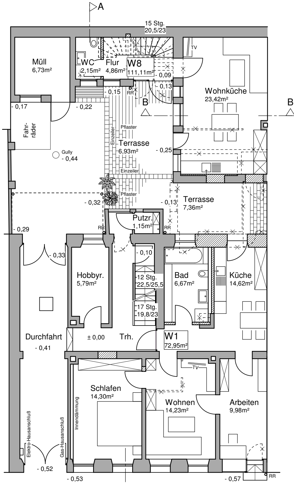
Erdgeschoss
